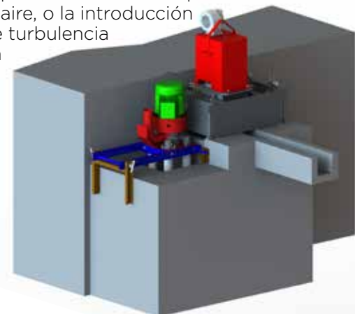
Sistema de Transferencia Launder MMEI Filtrada con Desgasificador Rotatorio
